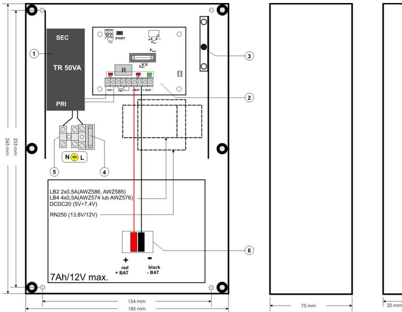
Rys.3. Widok zasilacza.
