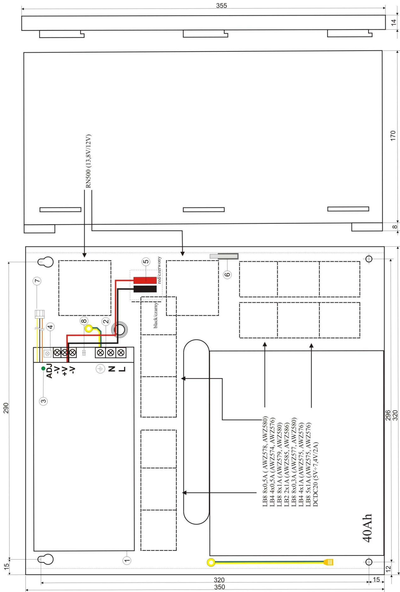
Rys.2. Widok zasilacza.
